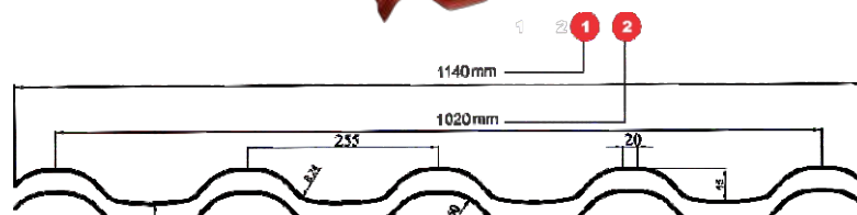
1 - Lățime totală 2 - Lățime utilă
